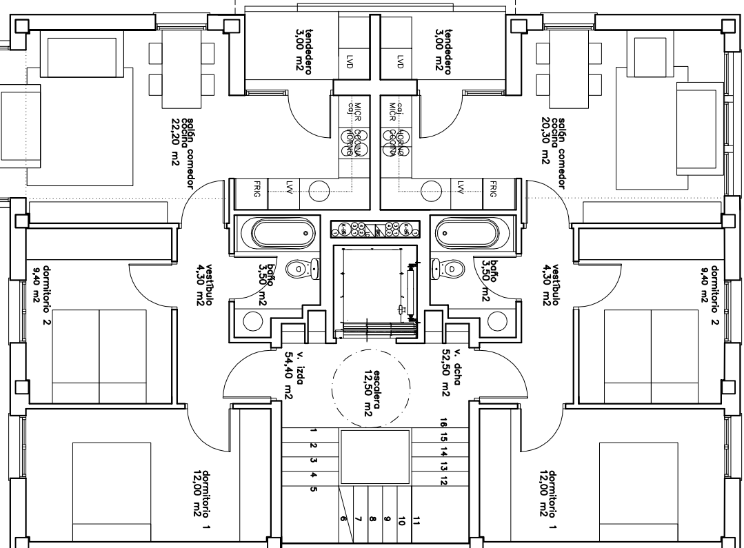
PLANTA PRIMERA
