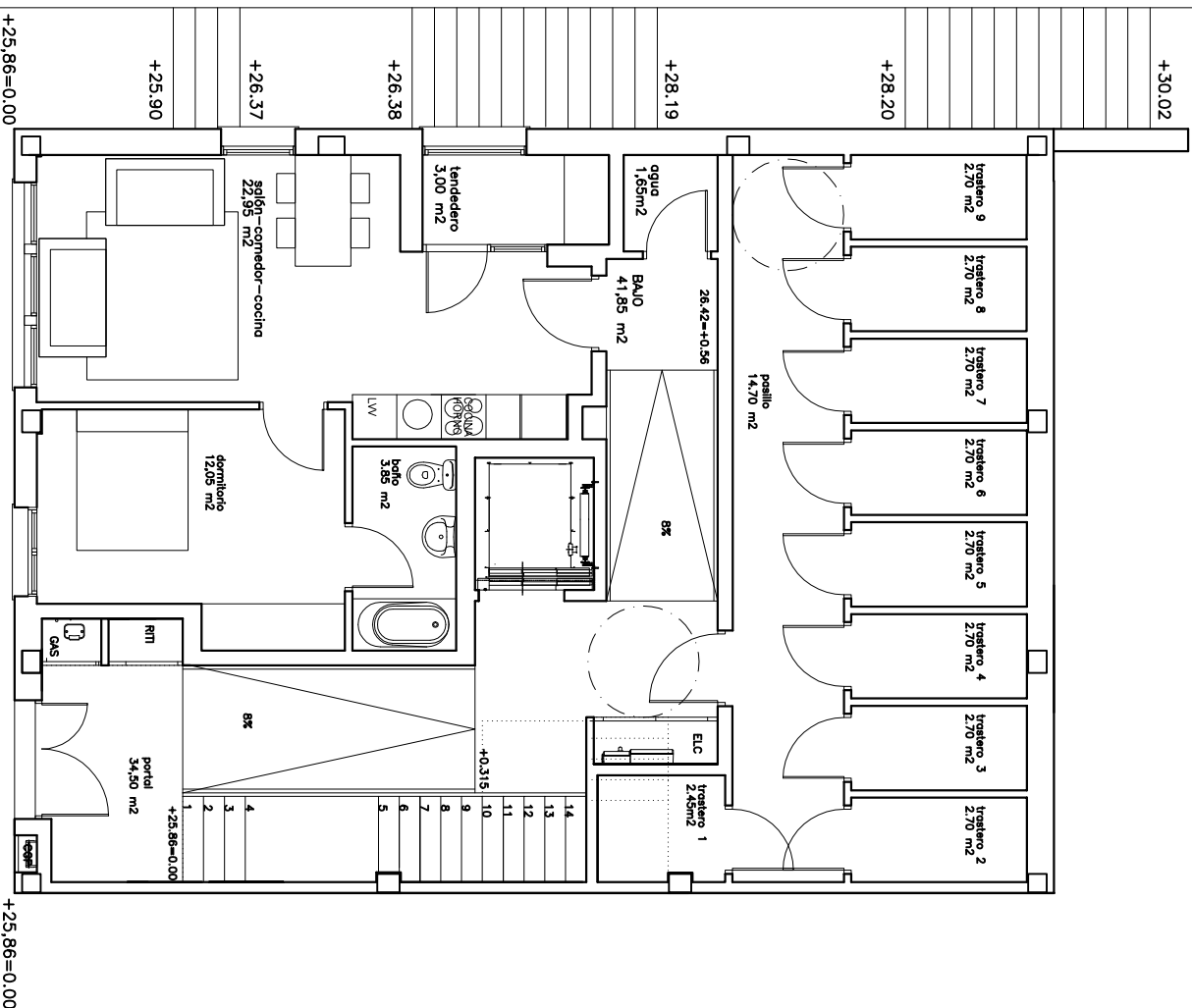
PLANTA BAJA
