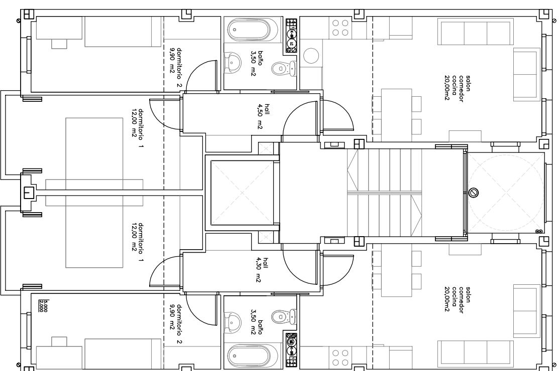
PLANTA 1ª (+3,50) PLANTA 2ª (+6,38) PLANTA 3ª (+9,26) PLANTA 4ª (+12,14)
